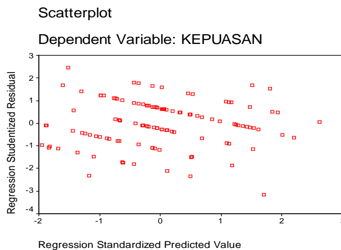
Gambar 3. Scaterplot Uji Heteroskedastisitas
